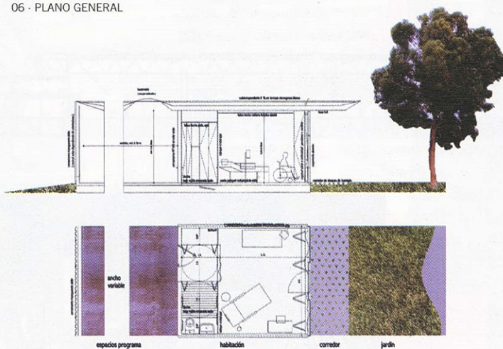
07 · SECCIÓN Y PLANTA
